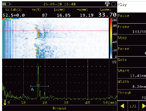
UT B-Scan
